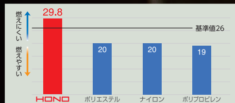
素材別燃焼指数 (LOI値)
